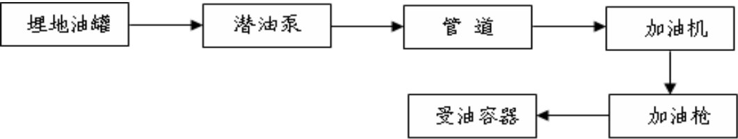
图 2.6-4 柴油加油机加油工艺流程图
