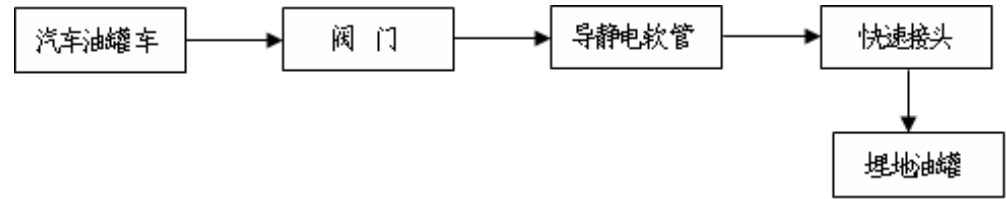
图 2.6-2 接卸柴油工艺流程图
