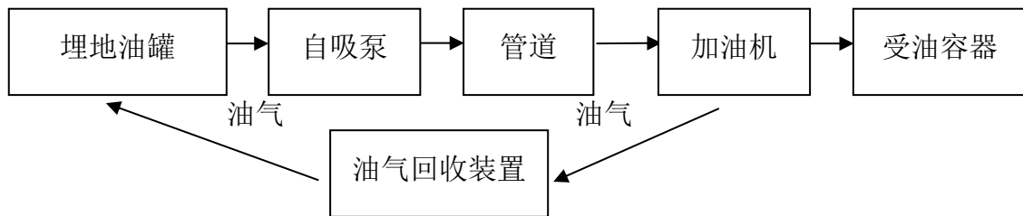
图 2.2-2 汽油加油工艺流程图
