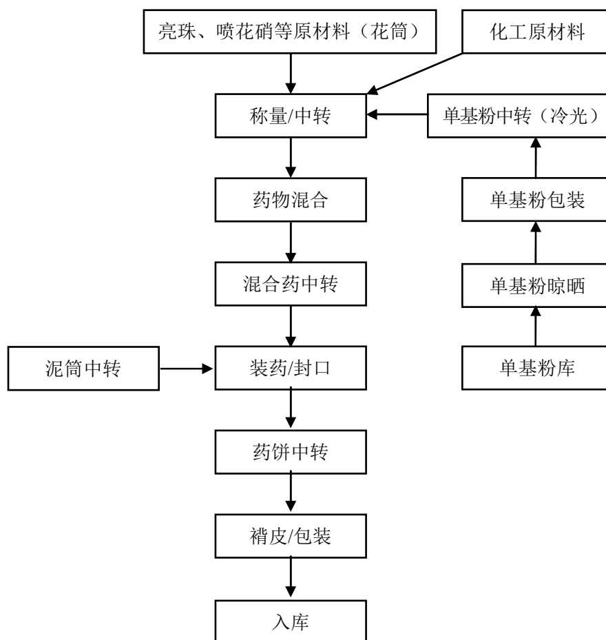
图 2.4-2 喷花类产品生产工艺流程图
