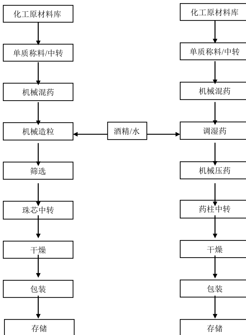
图 2.4-5 烟火药（亮珠、药柱）生产工艺流程
