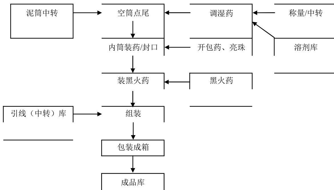
图 2.4-4 小礼花（内筒型）产品生产工艺流程图
