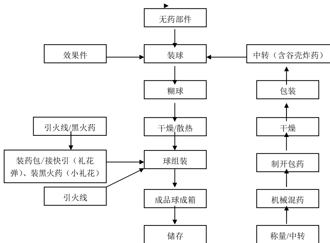
图 2.4-3 礼花弹/小礼花（球型）产品生产工艺流程图
