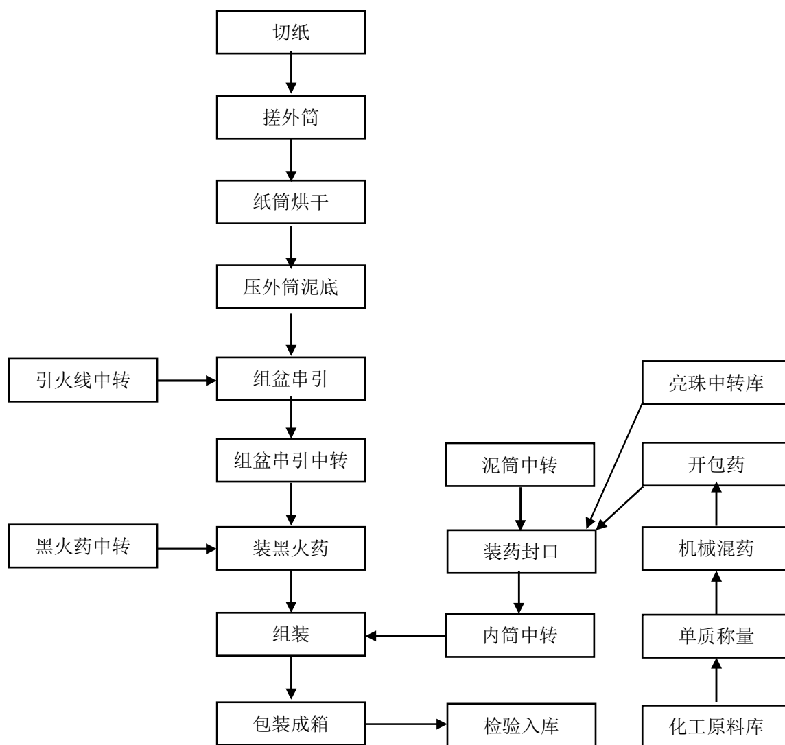
图 2.4-1 组合烟花类生产工艺流程图
