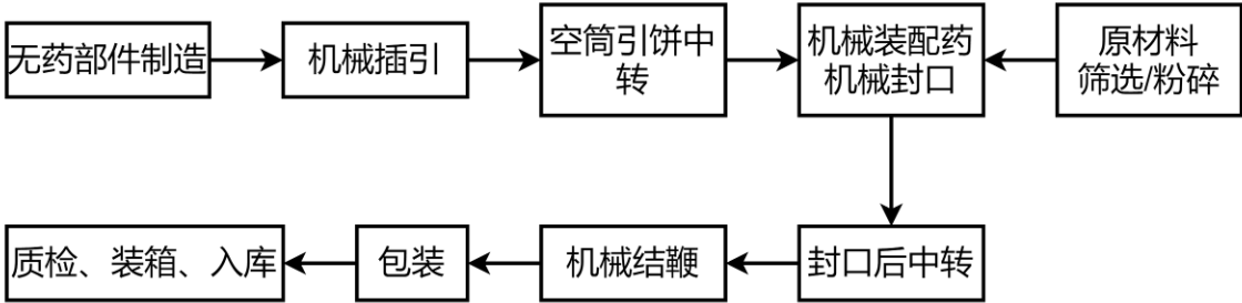
图 2-1：爆竹生产（插引）工艺流程
