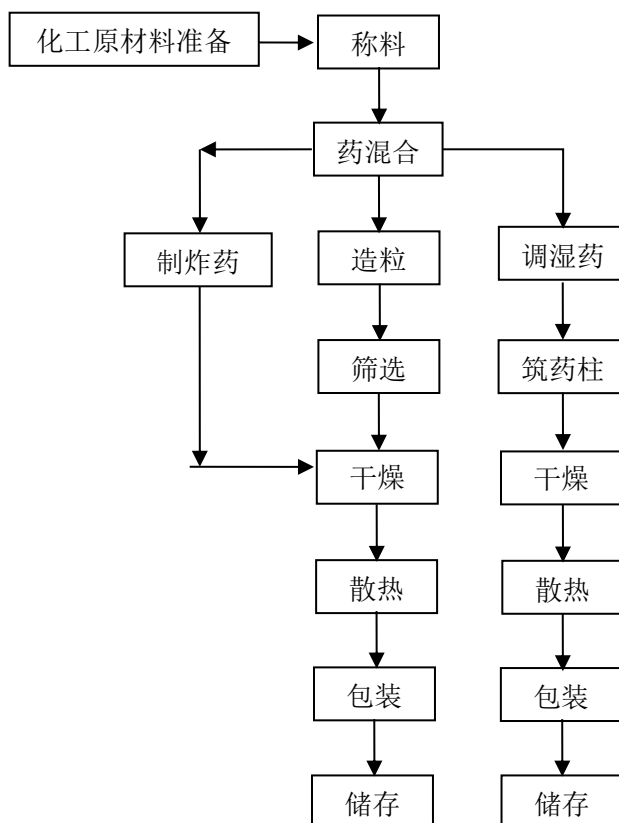
图 2.4-1 亮珠、炸药、药柱生产工艺流程图
