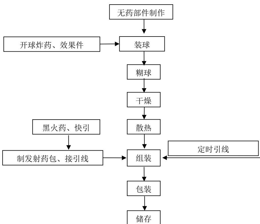
图 2.4-2 礼花类（礼花弹含球型小礼花）产品生产工艺流程图
