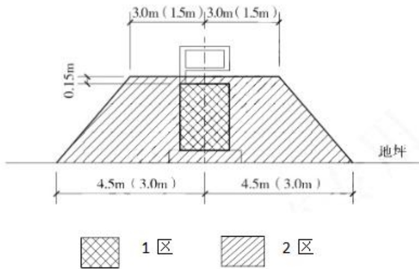
图3.10-2 汽油加油机爆炸危险区域划分
