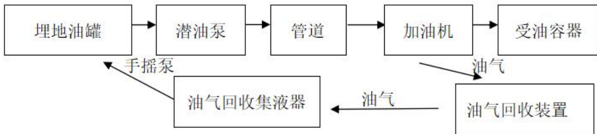
图 2.4-2 汽油加油工艺流程图
