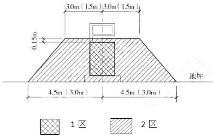
图 3.14-2 汽油加油机爆炸危险区域划分
